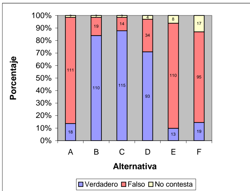
Figura 14.- Distribución de frecuencias para la cuestión número 3.
