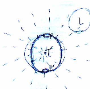
Figura 10.- La Tierra y líneas de puntos a modo de líneas de campo gravitacional en el que se incluye la Luna.
