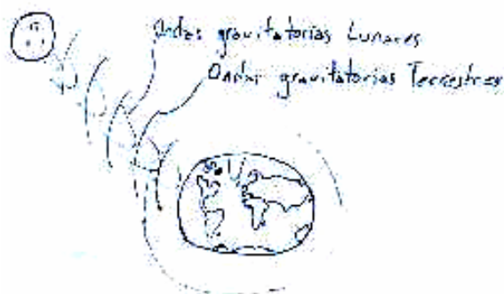
Figura 6.- La Tierra sigue el esquema del globo terrestre, la Luna guarda connotaciones "reales" en los cráteres y la interacción queda esquematizada por frentes de onda provenientes de cada cuerpo (R1.32).
