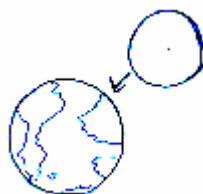
Figura 11.- La interacción entre la Tierra y la Luna ilustrada como una atracción terrestre (R1.15).
