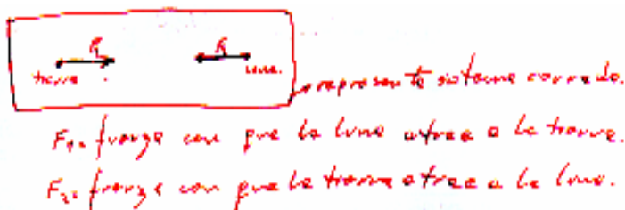
Figura 5.- La Tierra y la Luna son representadas por sendos puntos materiales. La interacción queda caracterizada por vectores fuerza (de igual magnitud y sentido contrario) aplicados en cada uno de los cuerpos celestes. (R1.4).
